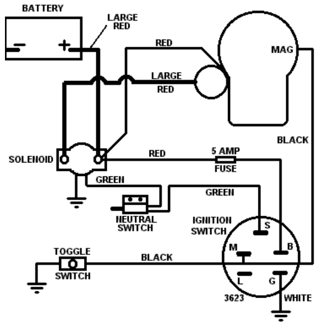
T44 12 VOLT START
